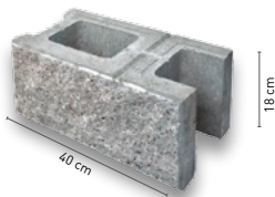
1 Pustak międzystupkowy 20×40×18 cm dwustronnie łamany
