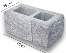
2 Pustak słupkowy dwoelementowy 20×40×18 cm czterostronnie łamany
